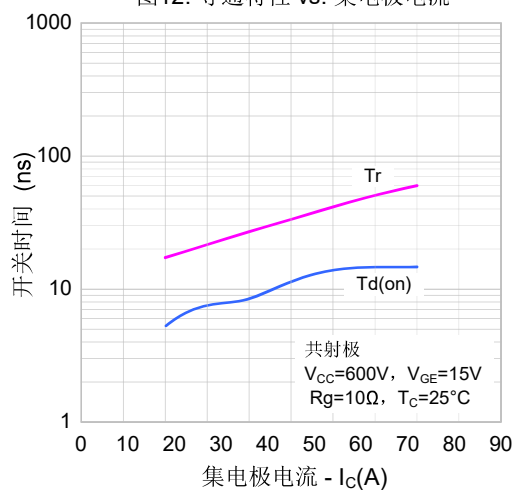
图12. 导通特性 vs. 集电极电流
